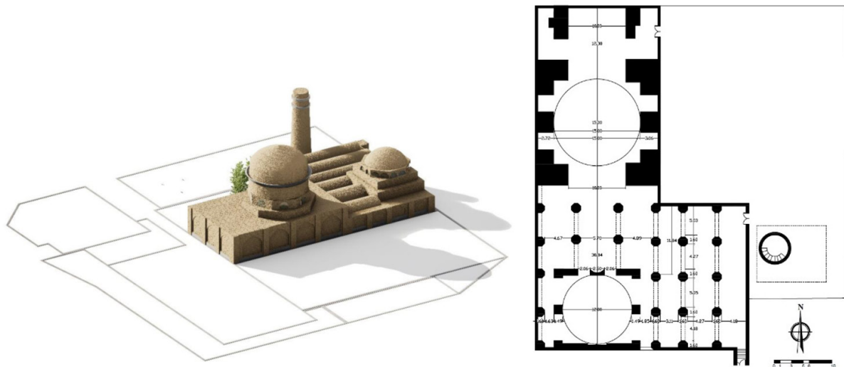
تصویر ۷. سمت چپ، پلان ترکمانی مسجد جامع کبیر تبریز طبق اسناد و شواهدات و بازآفرینی مسجد گسترش یافته با گنبد شمالی، مسجد جامع کبیر تبریز در دوره ترکمانی آق‌قویونلوها (مأخذ: نگارندگان)
