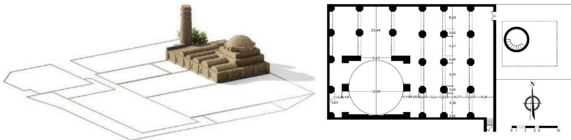
تصویر ۵. پلان سلجوقی مسجد جامع کبیر تبریز طبق اسناد و شواهدات و بازآفرینی مسجد با گنبد افزوده شده مسجد جامع کبیر تبریز در دوره سلجوقی (مأخذ: نگارندگان)
