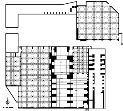
تصویر ۱۰. سمت چپ، پلان قاجار مسجد جامع کبیر تبریز طبق اسناد و شواهدات و بازآفرینی مجموعه مسجد جامع گسترش یافته در دوره قاجار (مأخذ: نگارندگان)
