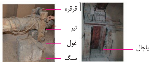
تصویر ۳. معرفی اجزای دستگاه تله سرکه در خانه‌ی بهشتیان (مأخذ: نگارندگان)
