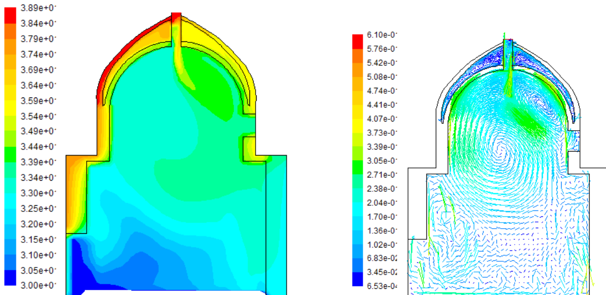
تصویر ۱۲. نمودار نمایش سطوح هم‌دما در مقطع عرضی ساختمان مینا در حالت گنبد همراه بادخان در رأس آن. در شرایط تابستان، روز. بر حسب درجه سانتی‌گراد. راست: نمودار سرعت خطوط جریان دما. چپ: نمودار نمایش سطوح هم‌دما (نرم‌افزار فلونت)
