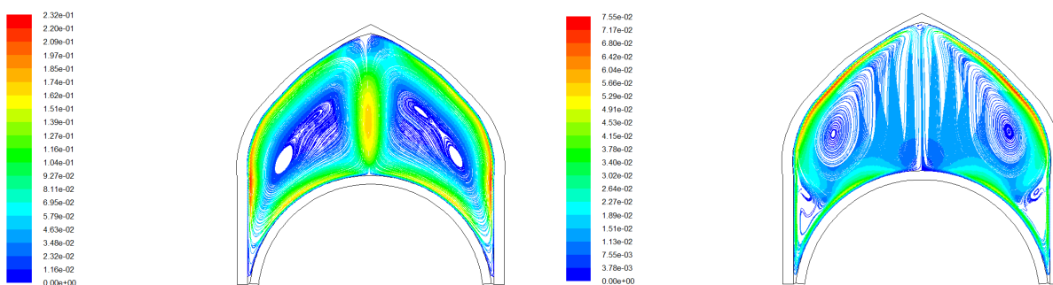
تصویر ۶. نمودار خطوط سرعت جریان در مقطع عمودی گنبد دو پوسته با ۳ متر لایه میانی هوا در راست: تابستان، روز (بین ۰،۰۰۳-۰،۷۵) چپ: زمستان، شب (بین ۰،۲-۰،۰۱). بر حسب متر بر ثانیه (نرم افزار فلوئنت)
