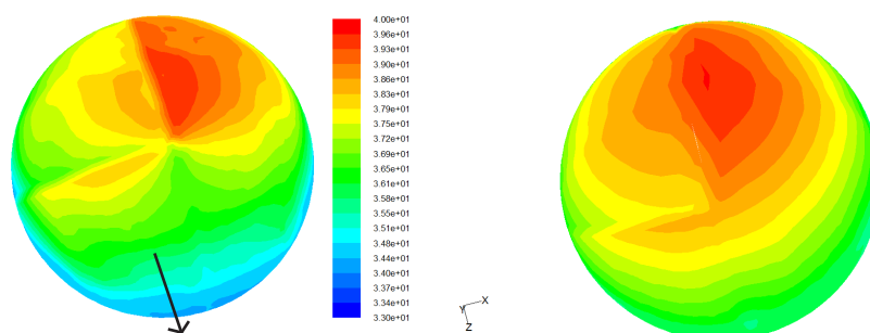
تصویر ۷. نمودار سطوح هم دما در سطح خارجی. راست: گنبد مبنا، چپ: گنبد قطاع کره متناظر با گنبد مبنا. در ساعت ۱۵ روز ۴ ژولای در کاشان. دما متغیر بین ۳۳-۴۰ درجه سانتی گراد. سمت شمال پایین است. (نرم افزار فلوئنت)
