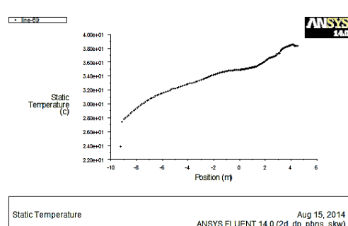
تصویر ۱۳. نمودار دما مکان در محور مرکزی مقطع عرضی ساختمان مینا در شرایط تابستان، روز. محور عمودی: دما بر حسب درجه سانتی‌گراد. محور افقی: مکان و نقطه صفر آن نماینده مرکز گنبد می‌باشد. راست: در حالت گنبد مینا. چپ: گنبد مینا همراه بادخان در رأس آن (نرم‌افزار فلونت)
