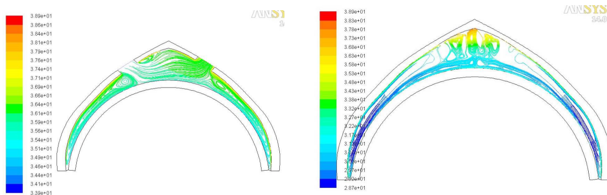
تصویر ۱۱. نمودار خطوط جریان دما در مقطع عمودی گنبد در تابستان، روز. راست: گنبد مینا. چپ: گنبد مینا با افزودن دریچه. بر حسب درجه سانتی‌گراد (نرم‌افزار فلوئنت)
